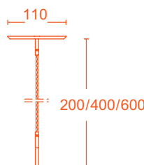
Hängevorrichtung
