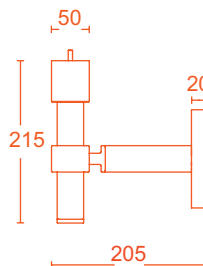
Wandhalterung
